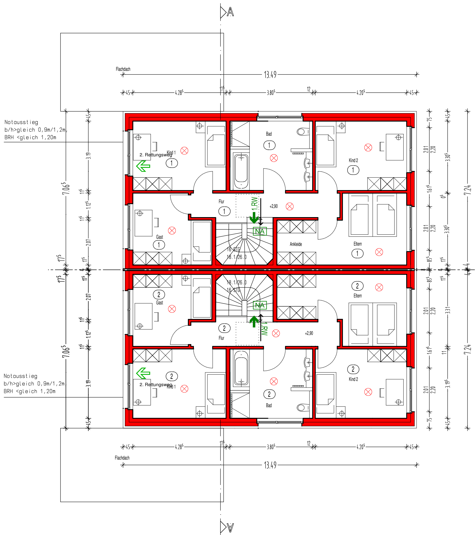
Dachgeschoss
